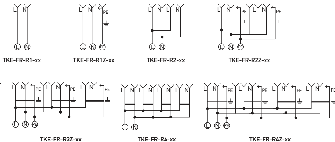
Рисунок 1. Электрические схемы розеток серии FREA (TOKOV™).
