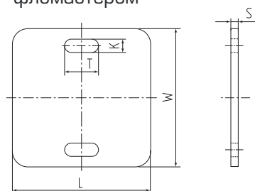
Конструкция бирок У-134
