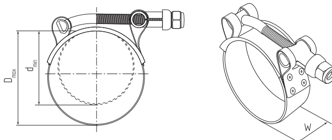
Конструкция силовых хомутов T-bolt ST/W2
