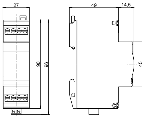
Габаритные размеры
