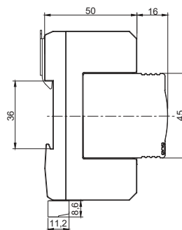
Габаритные размеры
