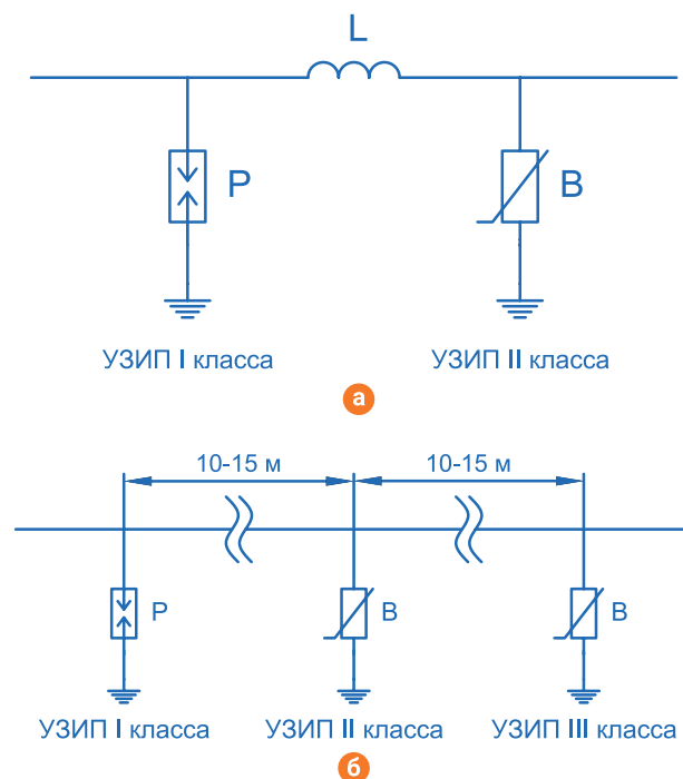
Рис. 10. Обеспечение селективной работы УЗИП:
