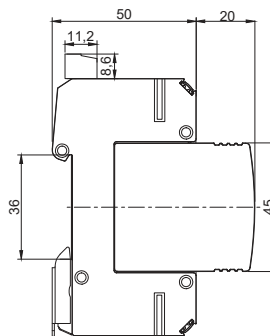
Габаритные размеры
