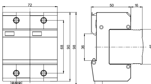
Габаритные размеры
