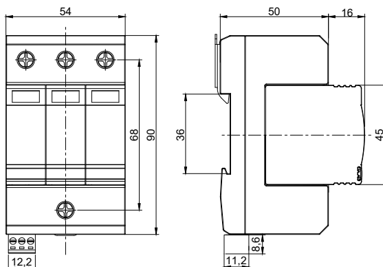
Габаритные размеры
