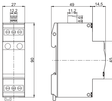
Габаритные размеры
