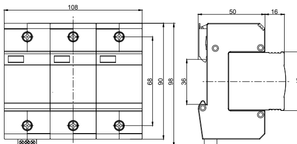
Габаритные размеры
