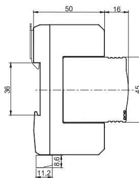
Габаритные размеры
