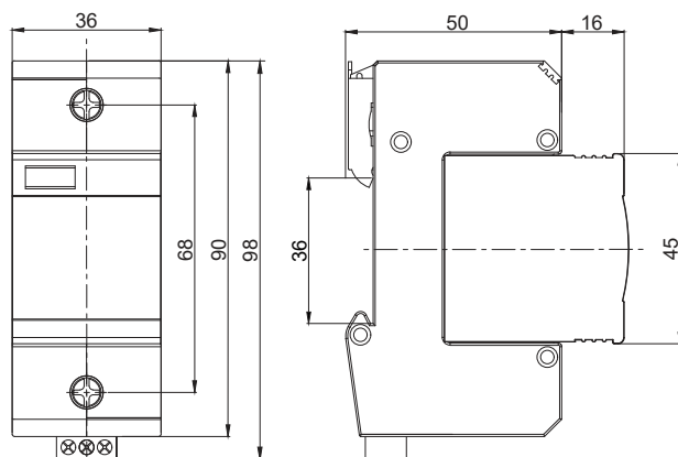
Габаритные размеры
