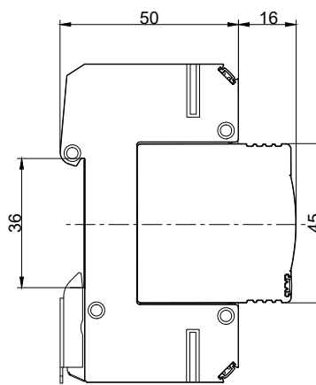
Габаритные размеры
