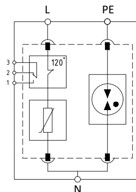
Принципиальная схема
