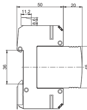
Габаритные размеры
