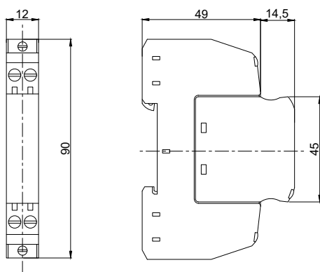
Габаритные размеры
