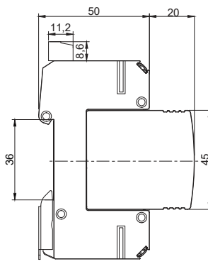
Габаритные размеры
