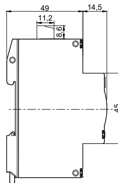
Габаритные размеры
