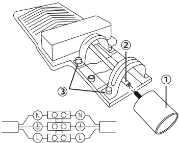
Рис. 1. Монтаж светильника
