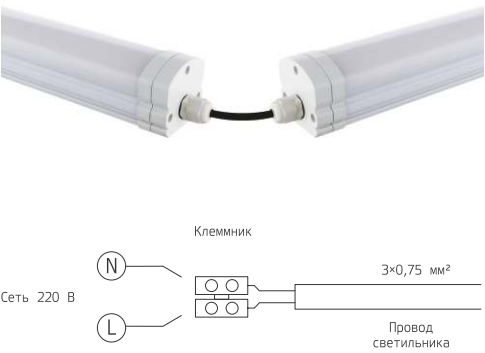
Рис. 1. Схема подключения светодиодного светильника Ultracompact к сети 220В
