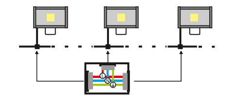
Рис. 1. Схема подключения прожектора к сети электропитания
