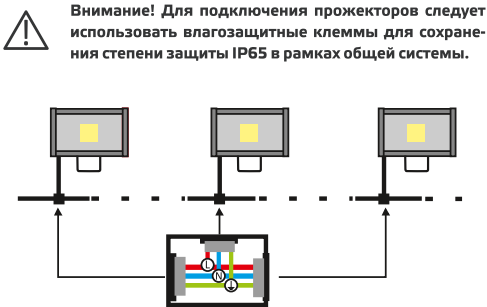
Рис. 1. Схема подключения прожектора к сети электропитания
