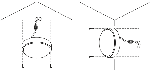
Рис. 2. Пример монтажа
