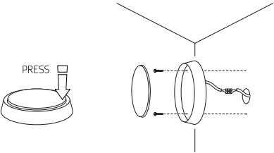
Рис. 1. Монтаж светильника
