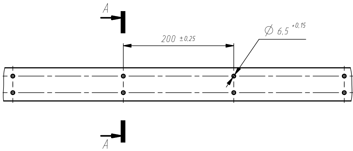
A-A (2:1)
