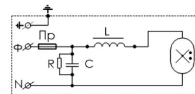
Рисунок 4 - Схема подключения к сети светильника PCY22
