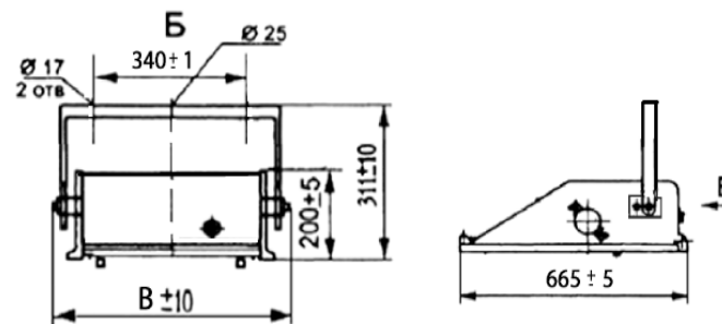
Рисунок 2 – Светильники серии ЖСУ22/PCY22/ГСУ22...004/005
