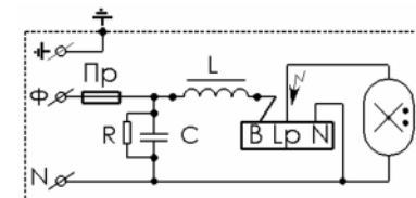
Рисунок 3 - Схема подключения к сети светильников ЖСУ22/ГСУ22
