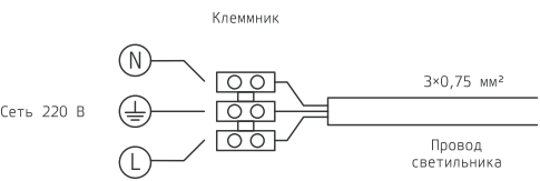
Рис. 1. Схема подключения светодиодного светильника к сети 220 В
