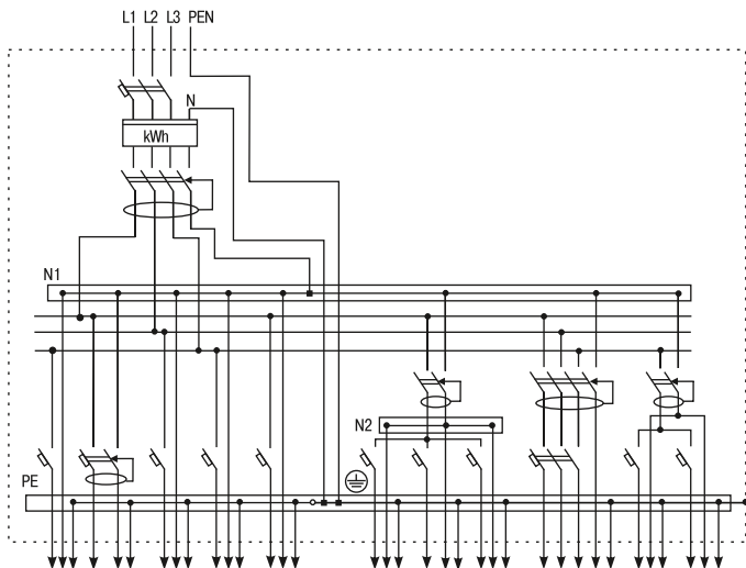
Рисунок 6 – Схема квартирного учетно-группового щитка (для коттеджа)
