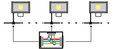
Рис. 1. Схема подключения прожектора к сети электропитания
