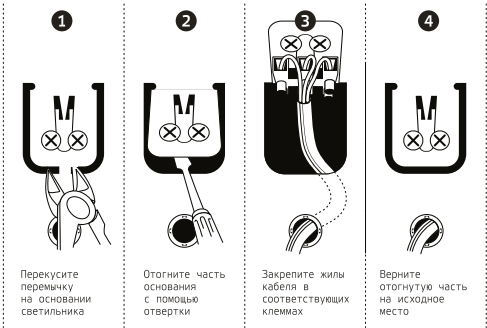
Рис. 3. Порядок монтажа
