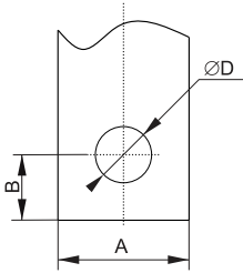
Рисунок 8а – шина для BA-35М
