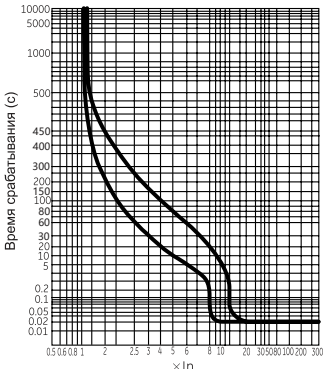
Рисунок 2а - Времятоковые характеристики выключателей BA88-32M с ln 32A Рисунок 2б - Времятоковые характеристики выключателей BA88-32M с ln>32A
