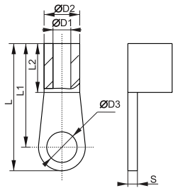
Рисунок 7б – Наконечник переходник для BA88-35M
