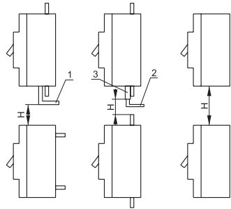
Рисунок 6 – Минимальные расстояния между двумя вертикально установленными выключателями.
