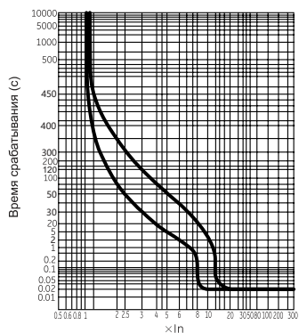
Рисунок 2в - Временноток-амперные характеристики выключателей ВА88-35М
