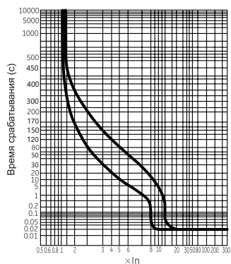
Рисунок 2г - Временноток-амперные характеристики выключателей ВА88-37М
