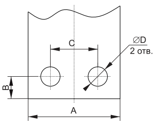
Рисунок 8б – шина для BA-35М
