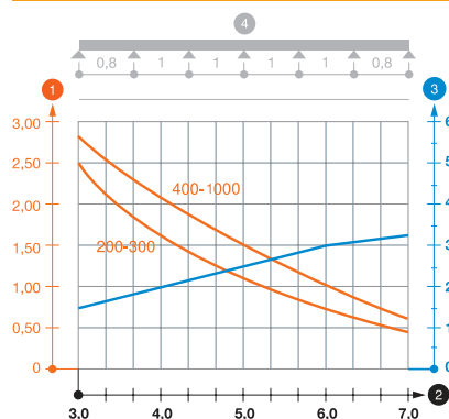
Диаграмма нагрузки на кабельный лоток лестничного типа для больших расстояний WKLG 110
