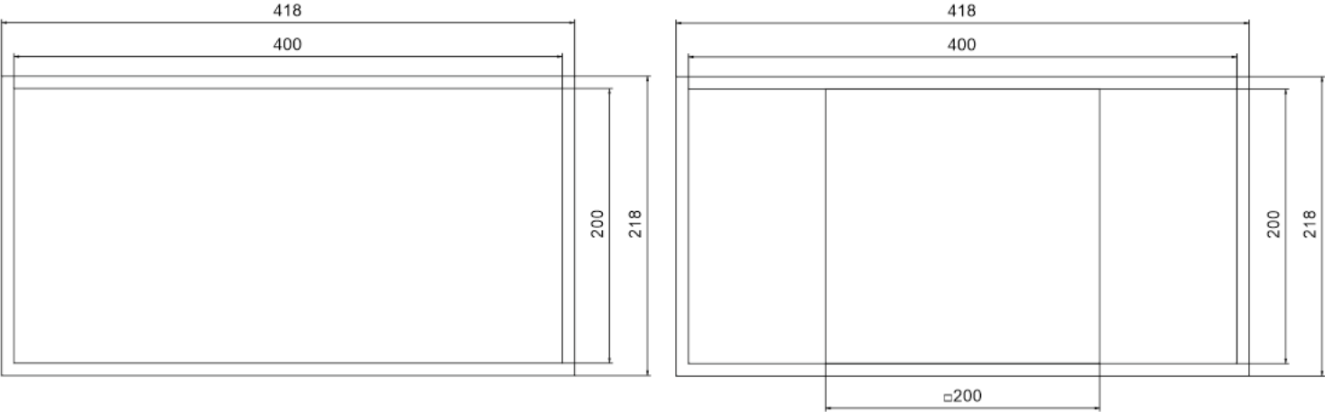
Приложение № 2. Габаритный чертёж.
