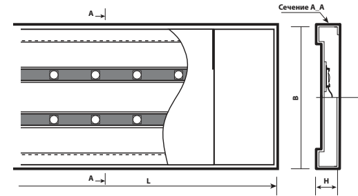
Рис 1. Светильник РРО-02
