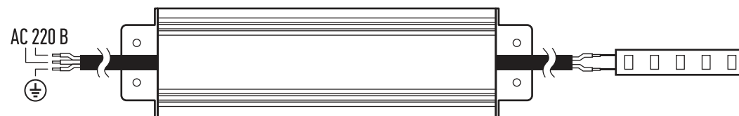
Схема подключения для моделей OD-P20-IP67-24V, OD-P30-IP67-24V, OD-P50-IP67-24V, OD-P60-IP67-24V
