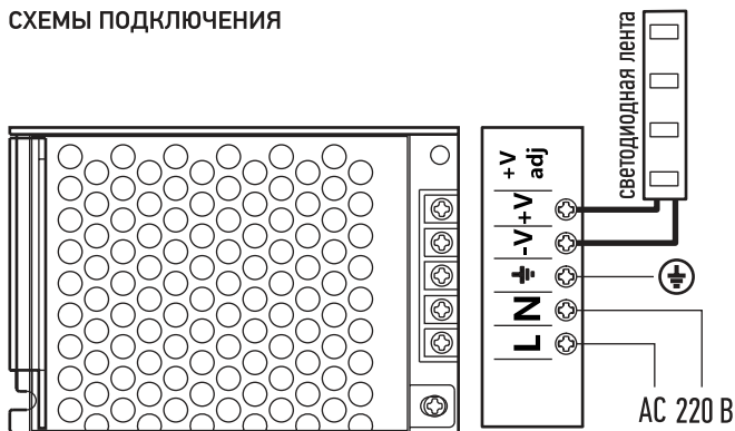
Схема подключения для моделей OD-P40-IP20-24V, OD-P60-IP20-24V
