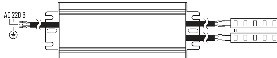
Схема подключения для модели OD-P200-IP67-24V
