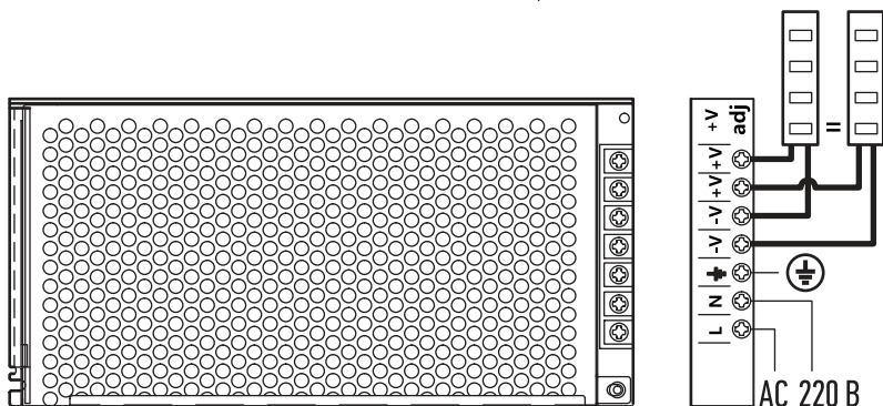
Схема подключения для моделей OD-P100-IP20-24V, OD-P120-IP20-24V, OD-P150-IP20-24V, OD-P200-IP20-24V
