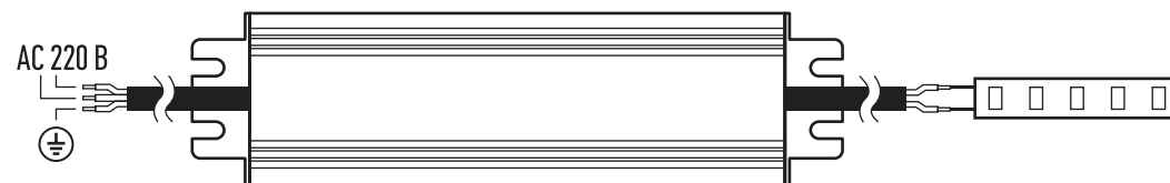
Схема подключения для моделей OD-P100-IP67-24V, OD-P150-IP67-24V
