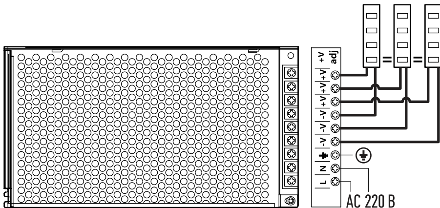
Схема подключения для модели OD-P250-IP20-24V
