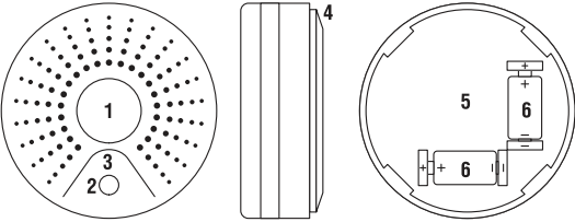
1 – корпус устройства; 2 – кнопка сброса/управления; 3 – светодиодный индикатор; 4 – задняя крышка; 5 – нижняя часть корпуса; 6 – элементы питания.
