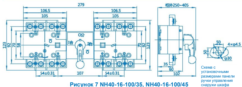
Рисунок 7 NH40-16-100/35, NH40-16-100/45
