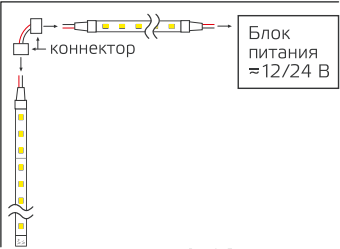
Рис. 1. Подключение коннектора
