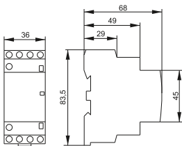
Контакторы KM20-22M AC, KM25-22M AC и KM20-40M AC
