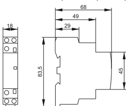
Контакторы KM20-20M AC и KM20-11M AC
