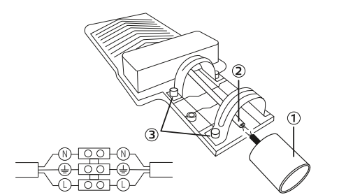
Рис. 1. Монтаж светильника
