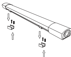
– Рисунок 1 – Установка при помощи монтажных скоб
