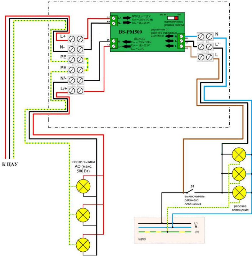
Приложение № 2 Схема подключения
