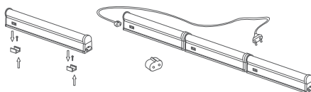
– Рисунок 2 – Установка при помощи монтажных скоб
