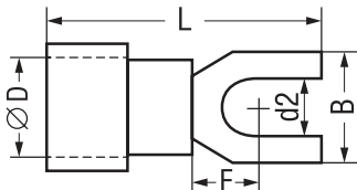
Рис. 3. Наконечники вилочные типа PTI
