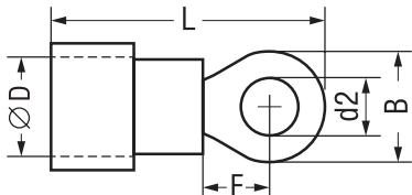
Рис. 2. Наконечники кольцевые типа RTI
