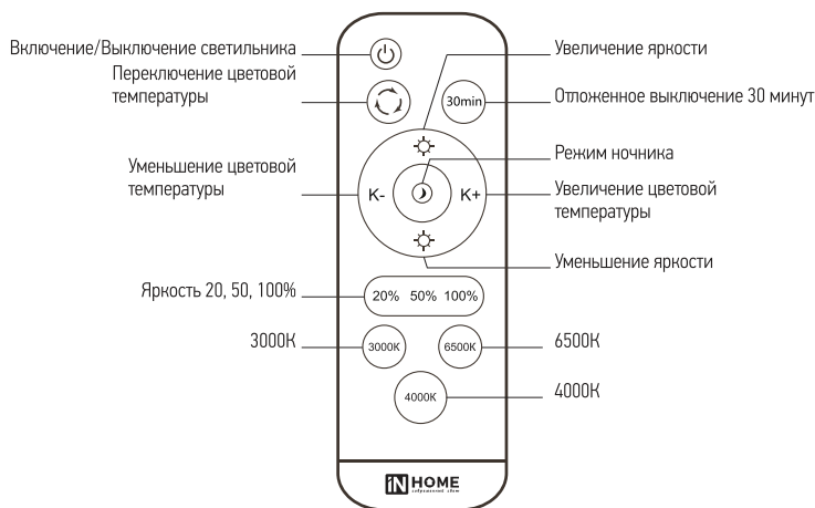
Рис. 1 Управление светильником
