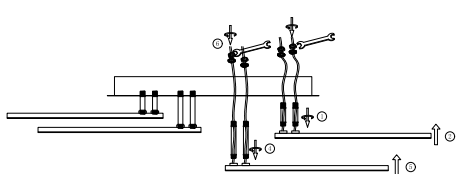
Монтажный чертеж потолочного светильника ELEGANT FLAME 120Вт
