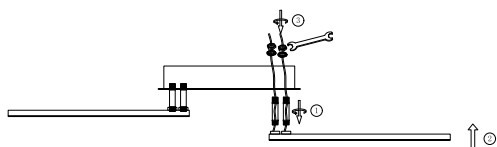
Монтажный чертеж потолочного светильника ELEGANT FLAME 90Вт
