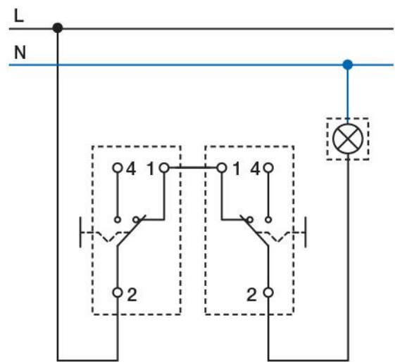
Принципиальная схема управления из 2 мест с помощью переключателя одинарного (требуется 2 переключателя 1E3140130x)
