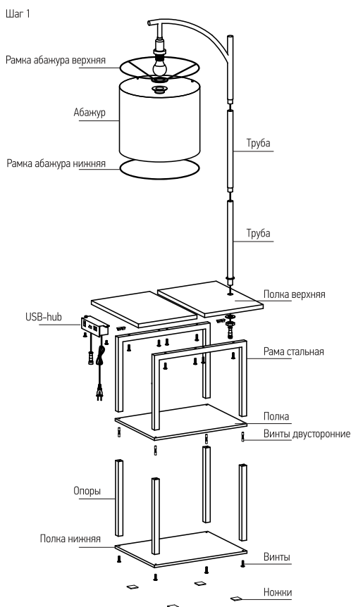
Рис. 1 Сборка светильника
