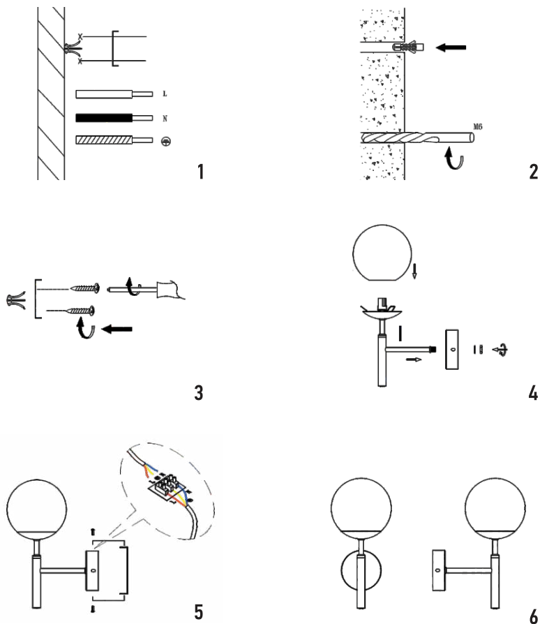
- Рис. 1. Схема подключения светильника
