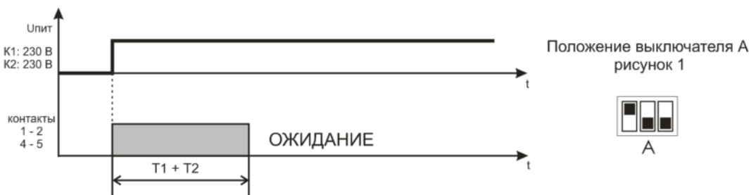
Рисунок 7 – Алгоритм работы Реле импульсное 2
