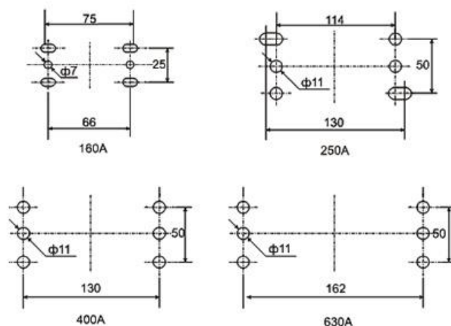
Рисунок 2. Установочные размеры.
