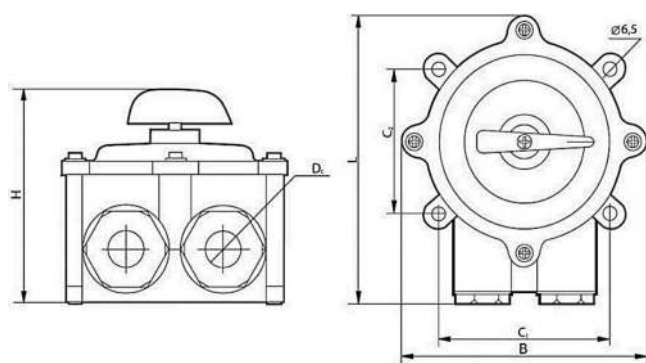
Рисунок 15. Габаритные и установочные размеры пакетных переключателей серии ПП. Исполнение в пластиковом корпусе. Степень защиты IP56. Способ крепления - основанием корпуса.
