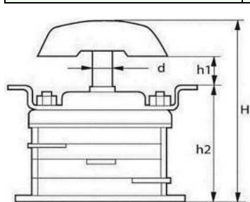
Рисунок 12. Габаритные и установочные размеры пакетных переключателей ППИ. Исполнение 1. Степень защиты IP00. Способ крепления - передней скобой.
