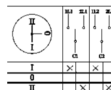
Пакетный переключатель ПП 2-полюсный на 2 направления
