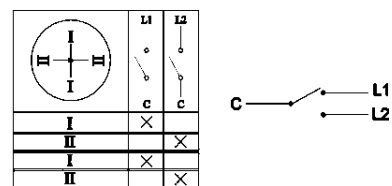
Пакетный переключатель ПП 1-полюсный 4С специального исполнения
