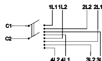
Пакетный переключатель ПП 2-полюсный на 4 направления
