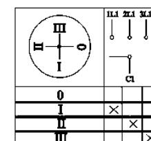
Пакетный переключатель ПП 1-полюсный на 3 направления
