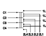
Пакетный переключатель ПП 4-полюсный на 2 направления
