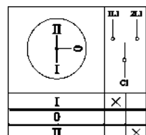
Пакетный переключатель ПП 1-полюсный на 2 направления
