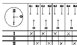
Пакетный переключатель ПП 4-полюсный на 2 направления
