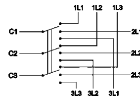
Пакетный переключатель ПП 3-полюсный на 3 направления
