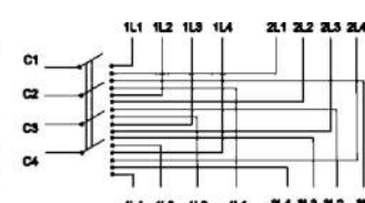
Пакетный переключатель ПП 2-полюсный на 4 направления
