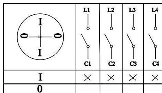
4-полюсный
