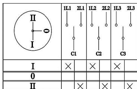
3-полюсный
