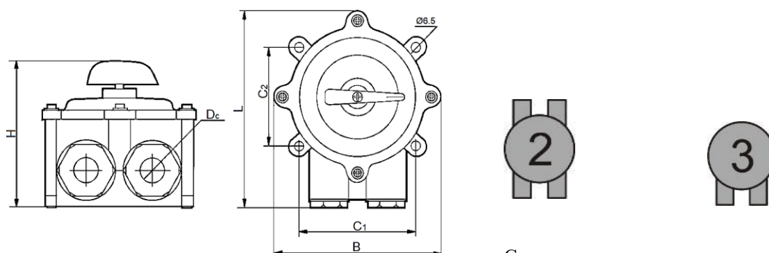
Схема расположения сальников
