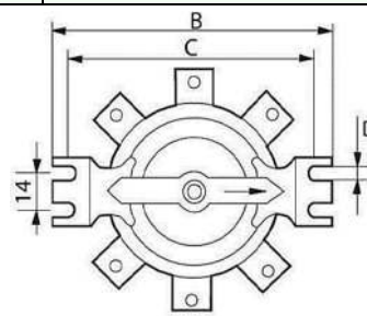
Рисунок 12. Габаритные и установочные размеры пакетных переключателей ПП. Исполнение 1. Степень защиты IP00. Способ крепления - передней скобой.
