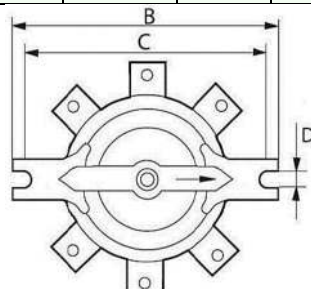
Рисунок 12. Габаритные и установочные размеры пакетных переключателей ПП. Исполнение 1. Степень защиты IP00. Способ крепления - передней скобой.
