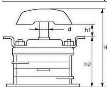
Рисунок 12. Габаритные и установочные размеры пакетных переключателей ПП. Исполнение 1. Степень защиты IP00. Способ крепления - передней скобой.
