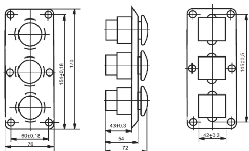
Рисунок 5. Габаритные и установочные размеры поста
