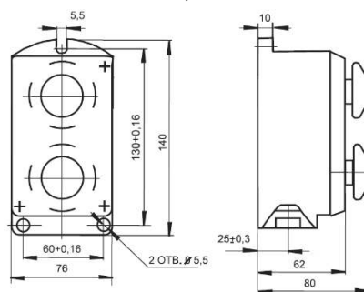
Рисунок 4. Габаритные и установочные размеры поста управления кнопочного ПКЕ 212-2; ПКЕ 222-2
