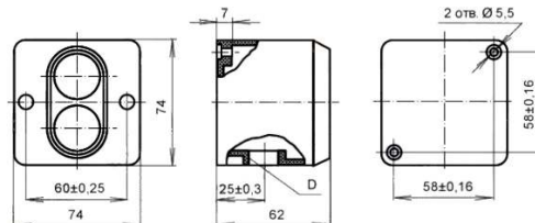
Рисунок 8. Габаритные и установочные размеры поста управления кнопочного ПКЕ 712; ПКЕ 722
