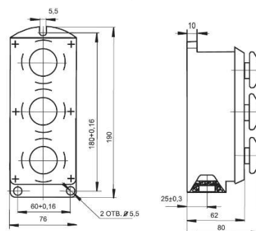
Рисунок 6. Габаритные и установочные размеры поста
