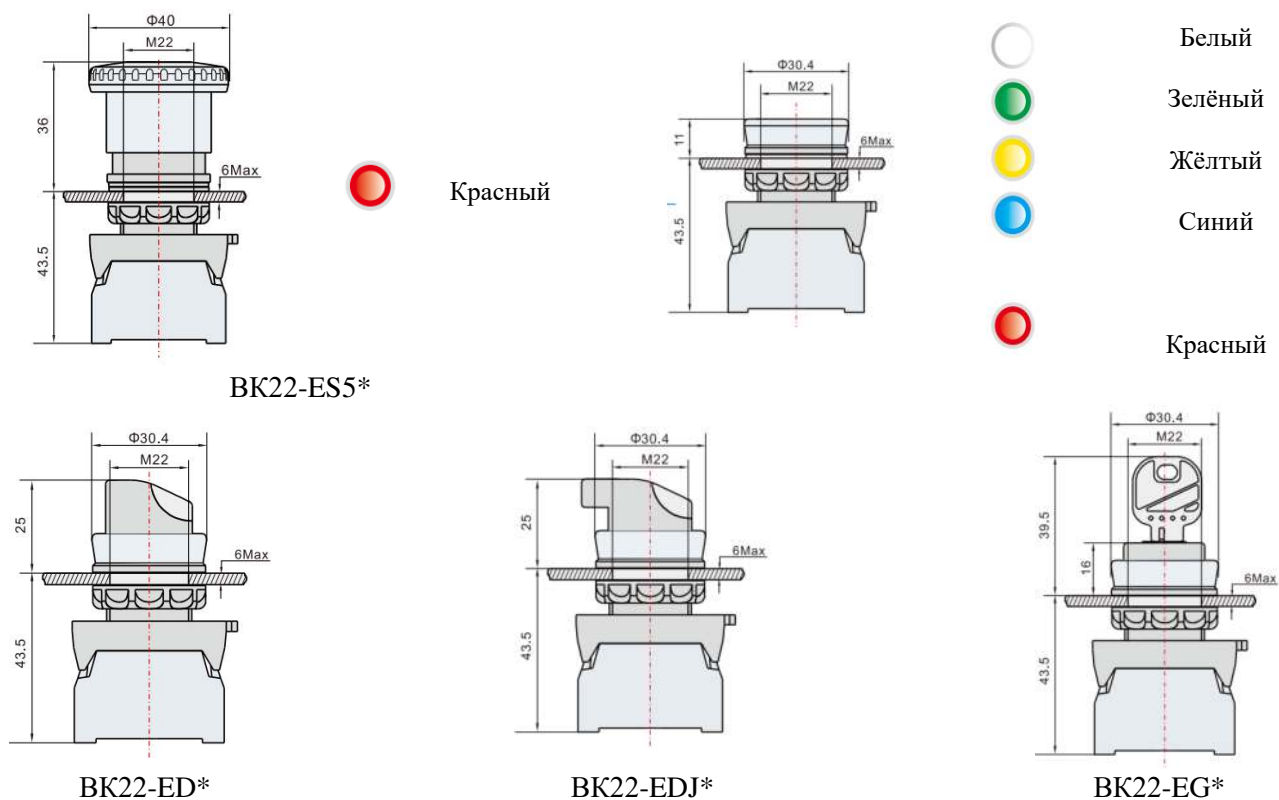
Рисунок 1. Выключатели, переключатели кнопочные серии BK22 IP65
