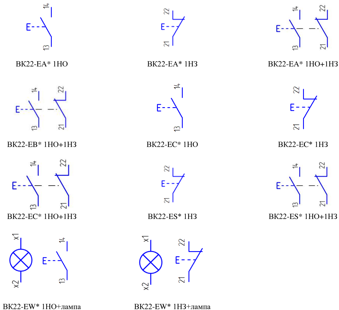
Рисунок 1. Выключатели, переключатели кнопочные серии BK22 IP65
