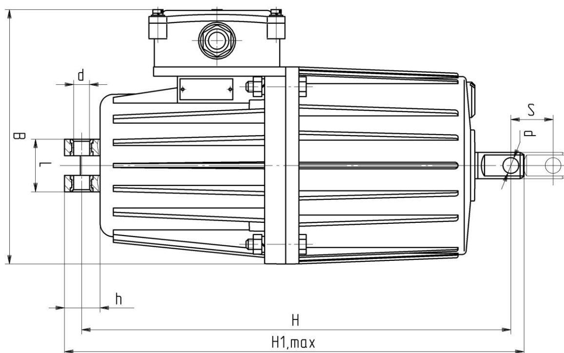
Рисунок. Габаритные и установочные размеры ТЭ
