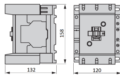
Рисунок 6. Контакторы LC1E120...160
