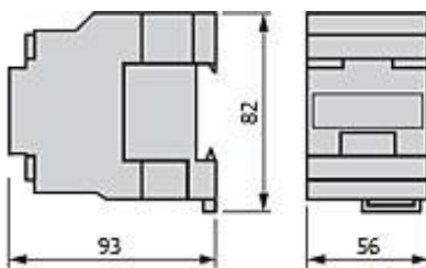
Рисунок 2. Контакторы LC1E25
