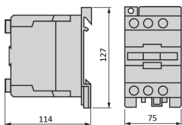
Рисунок 4. Контакторы LC1E40...65
