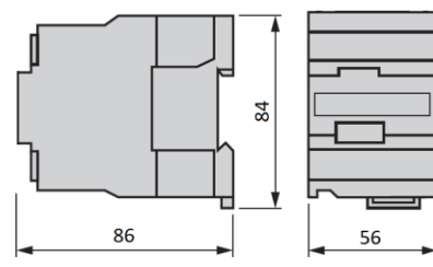
Рисунок 3. Контакторы LC1E32...38
