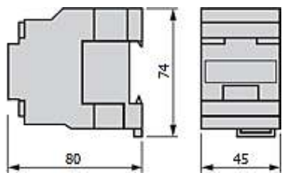
Рисунок 1. Контакторы LC1E06...18
