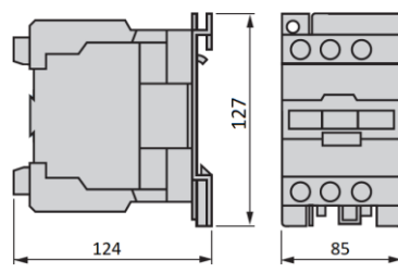
Рисунок 5. Контакторы LC1E80...95
