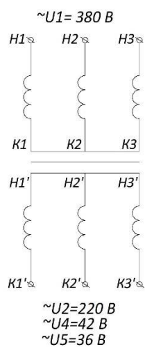
Рисунок 2. Принципиальные электрические схемы трансформаторов ТСЗИ
