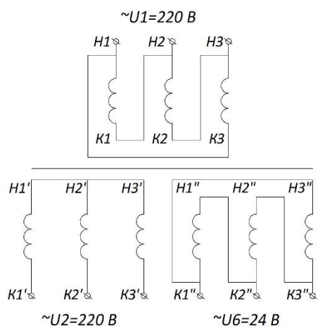
ТС3И-(1,6-2,5-4,0)-220/220;24
