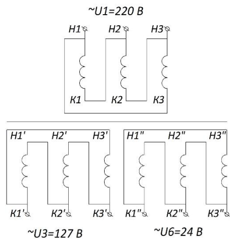
ТС3И-(1,6-2,5-4,0)-220/127;24
