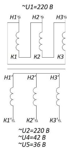
Рисунок 2. Принципиальные электрические схемы трансформаторов ТСЗИ
