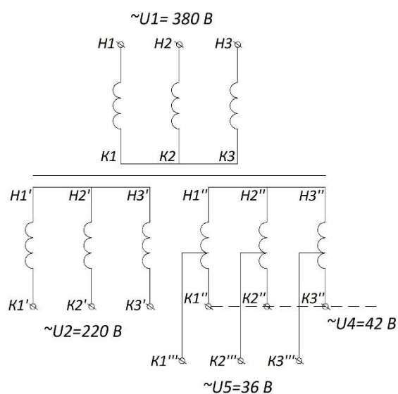
ТСЗИ-(1,6-2,5-4,0)-380/220;42;36
