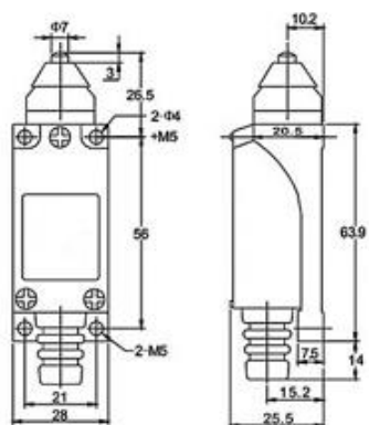
Рис. 1. ВП 25-2110 (толкатель)
