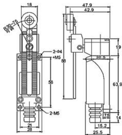
Рис. 4. ВП 25-2143/45 (рычаг с роликом, регулируемый по длине)
