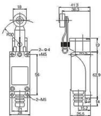
Рис. 3. ВП 25-2116/18 (рычаг с роликом)
