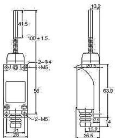
Рис.7. ВП 25-2107 (рычаг пружинный с пластиковым наконечником)
