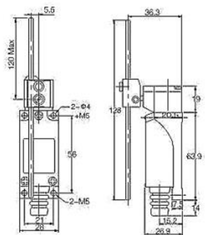
Рис.8. ВП 25-2153 (круглый стальной рычаг, регулируемый по длине)
