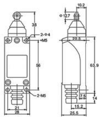
Рис. 2. ВП 25-2102 (толкатель с роликом)
