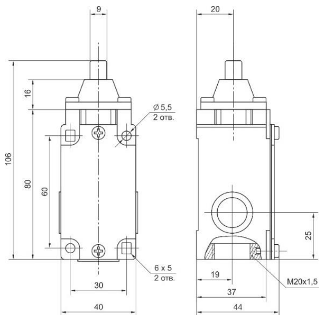
толкатель
