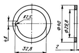
Рисунок 4. Размеры установочных резиновых прокладок
