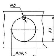
Рисунок 3. Размеры установочного отверстия в панели для установки переключателей
