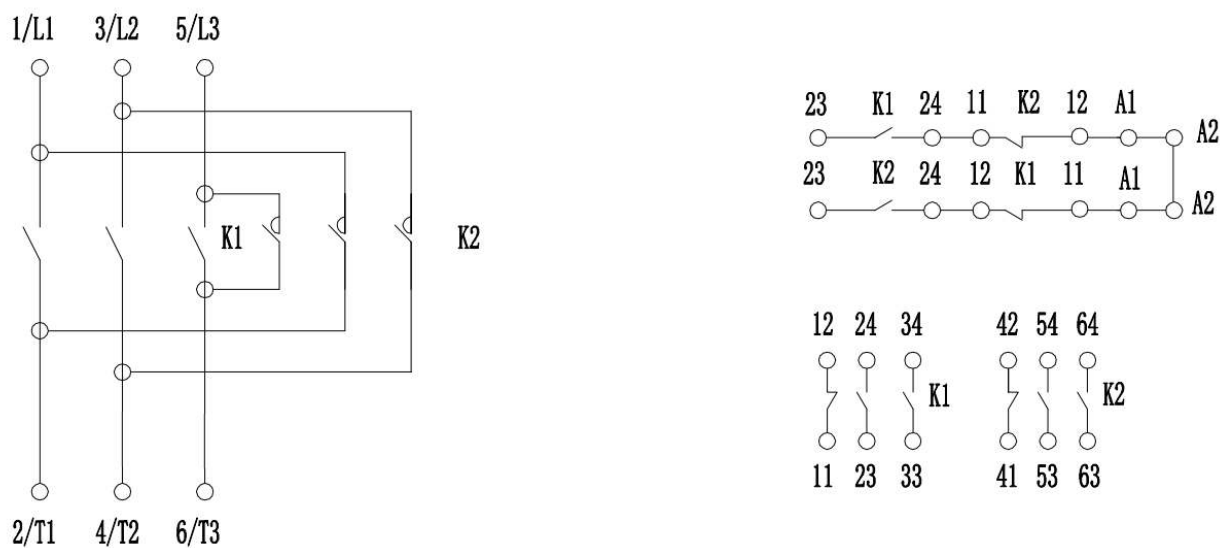
Рисунок 5. Принципиальная электрическая схема реверсивного пускателя ПМ12 315-630А
