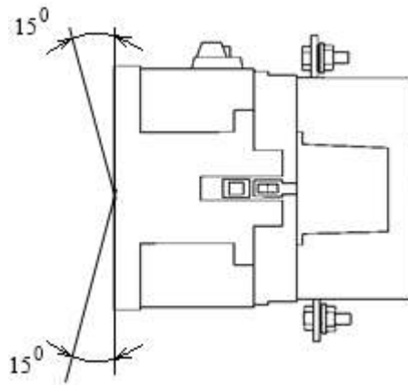
Рисунок 3. Рабочее положение пускателя
