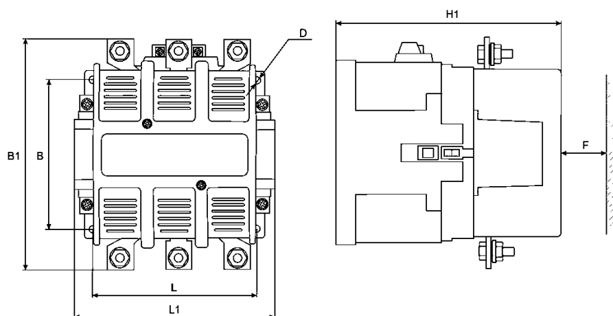
Рисунок 1. Пускатель нереверсивный типа ПМ12 315-1250А. Степень защиты - IP00
