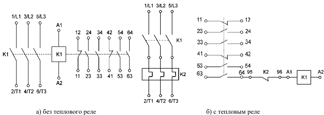
Рисунок 4. Принципиальная электрическая схема пускателя ПМ12 315-1250А
