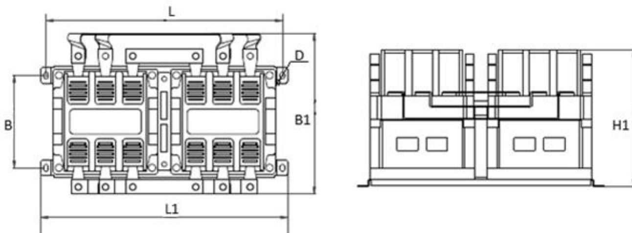
Рисунок 6. Пускатель реверсивный типа
