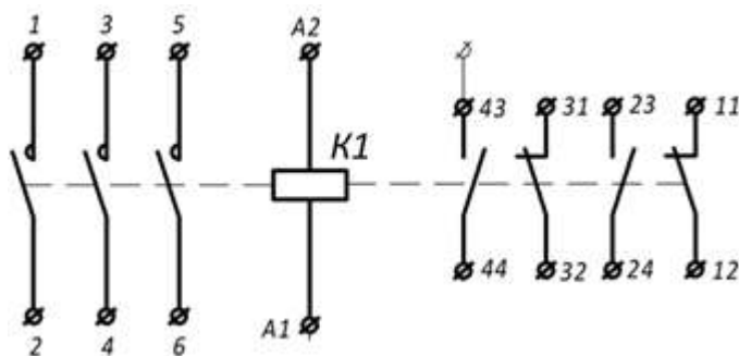
Рисунок 1. Схема пускателя без теплового реле
