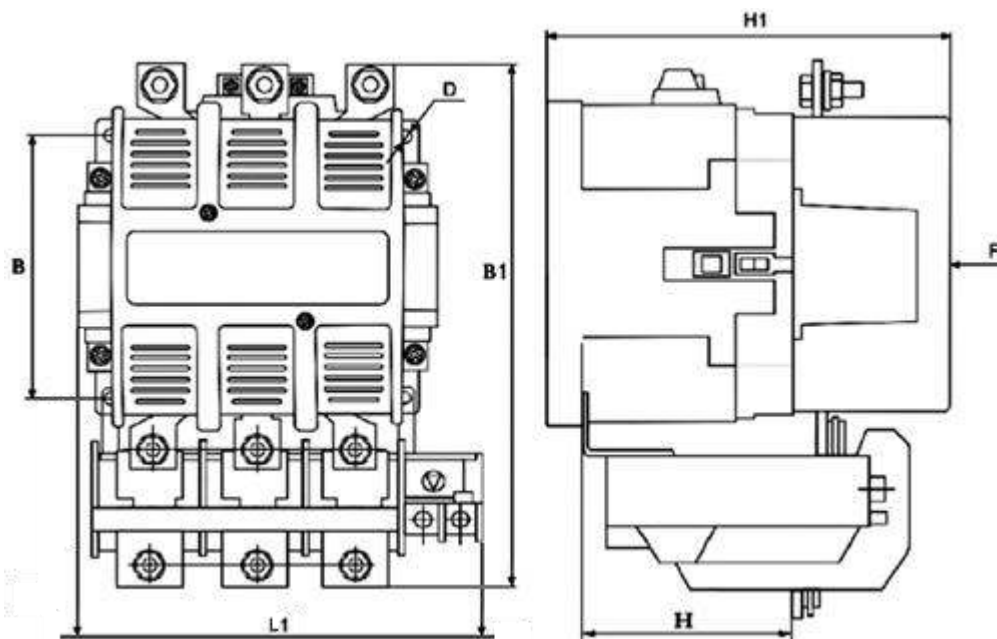
Рисунок 5. Пускатель нереверсивного типа с тепловым реле
