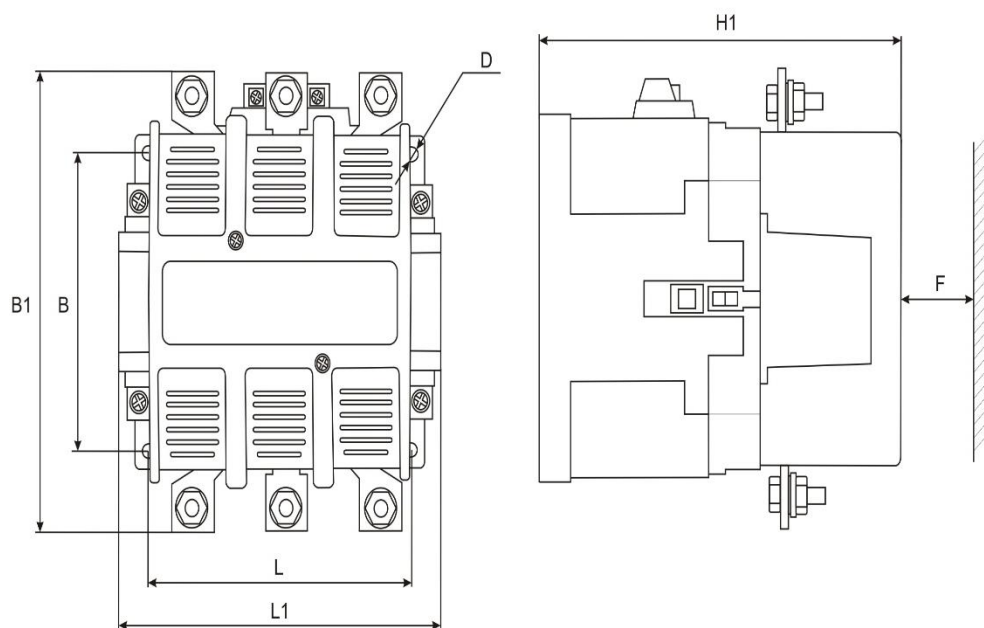
Рисунок 4. Пускатель нереверсивный типа
